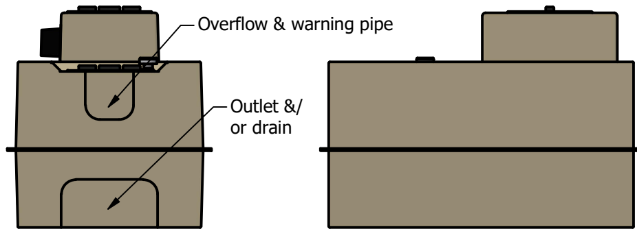
ELEV A
