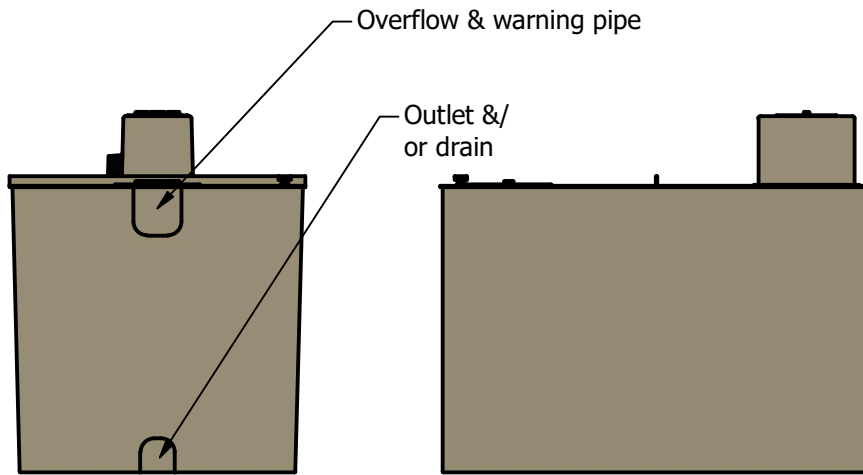
ELEV A
